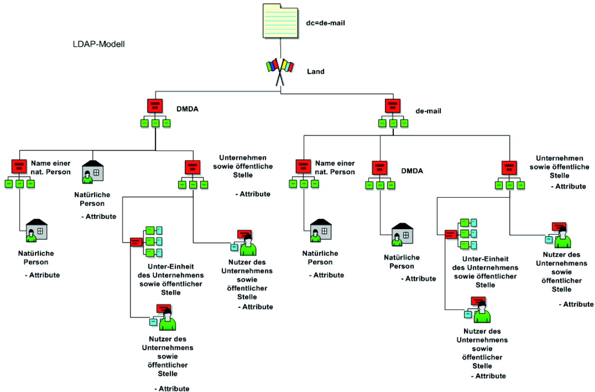
Abbildung 1: LDAP-Modell
