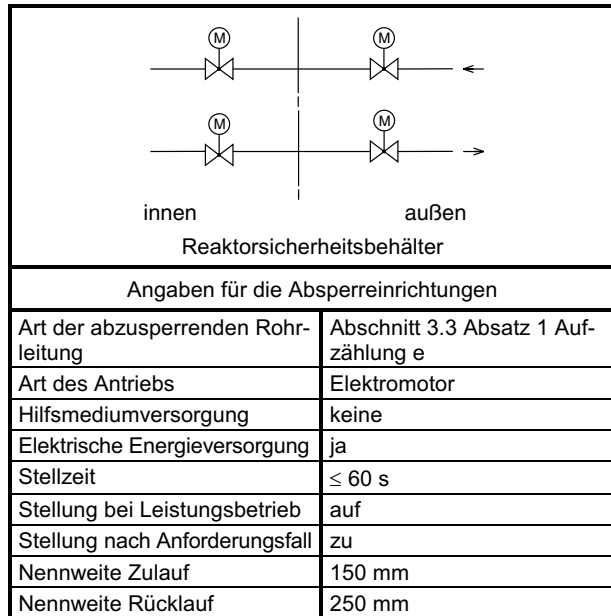
Bild A-9: Beispiel einer Anordnung von Absperreinrichtungen für die Ölversorgung der Hauptkühlmittelpumpe beim Siedewasserreaktor
