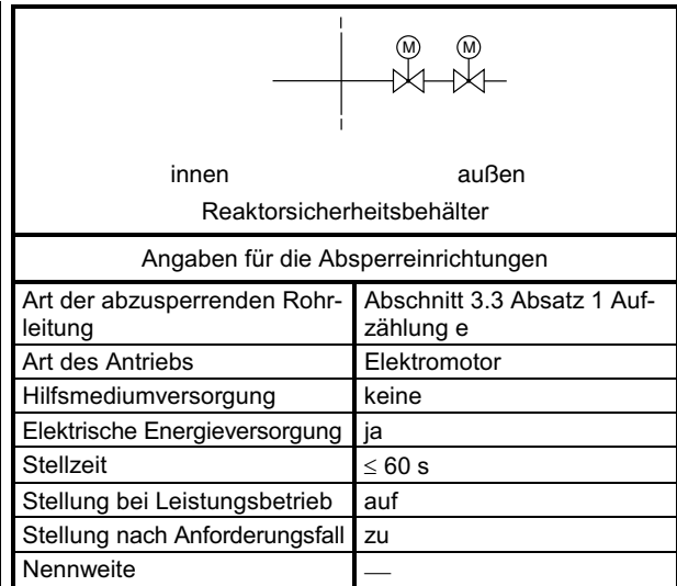
Bild A-11: Beispiel einer Anordnung von Absperreinrichtungen für ein System, das außerhalb des Reaktorsicherheitsbehälters nicht gegen den Auslegungsdruck des Reaktorsicherheitsbehälters ausgelegt ist
