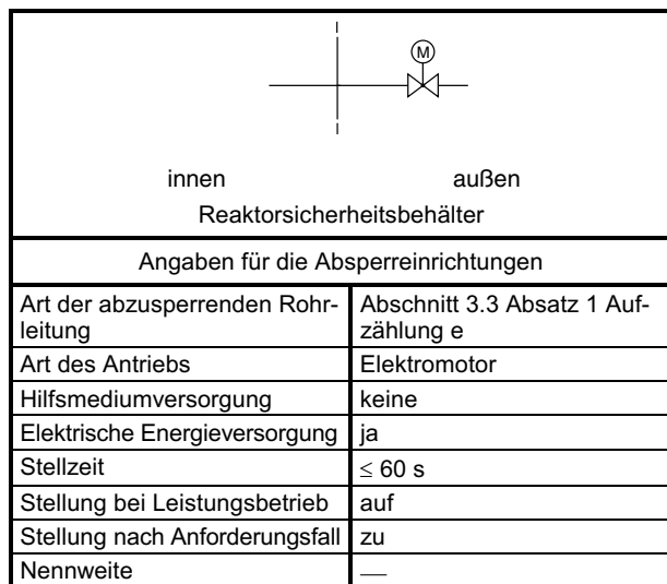
Bild A-10: Beispiel einer Anordnung von Absperreinrichtungen für ein System, das außerhalb des Reaktorsicherheitsbehälters gegen den Auslegungsdruck des Reaktorsicherheitsbehälters ausgelegt ist
