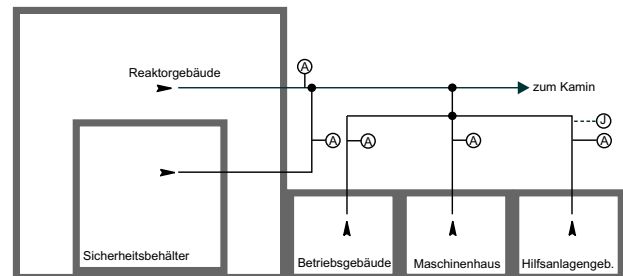
Bild 3-1: Beispiel einer Raumluftüberwachung beim DWR
