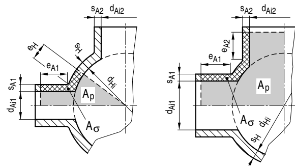
Bild A 3.1-10: Gehäusekörper
