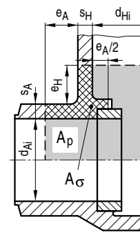
Bild A 3.1-10: Gehäusekörper
