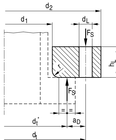
Bild A 2.9-6: Losflansch
