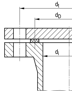
Bild A 2.6-2: Runde ebene Platten mit zusätzlichem Randmoment
