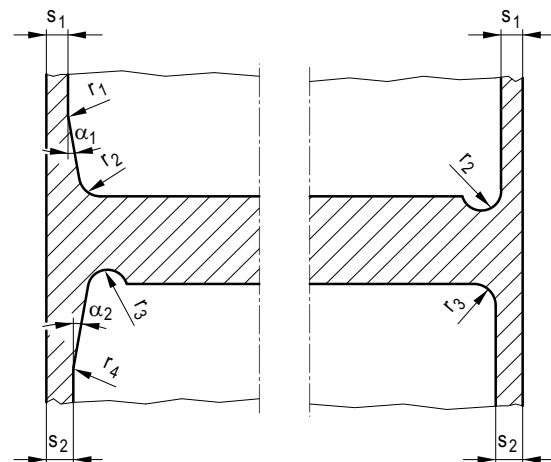
Bild 5.3-1: Beispiele für Rohrboden-Ausführungsformen
