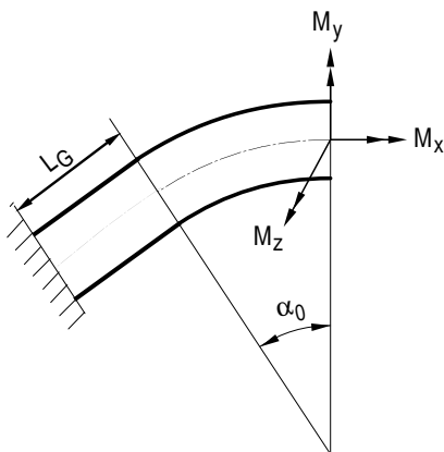
Bild 8.4-9: Definition der Momentenrichtung
