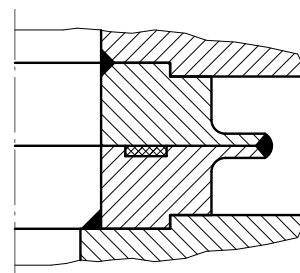
Bild 5.2-2: Beispiele für HV- und DHV-Nähte bei Anschweißungen
