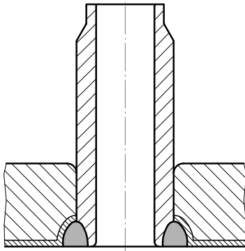
Bild 5.2-4: Beispiel für Anschweißungen an austenitische Schweißplattierungen
