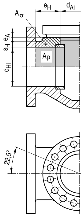
Bild A 3.1-7: Gehäusekörper
