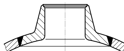
Bild 5.2-8: Beispiele für Stutzen-Ausführungsformen
