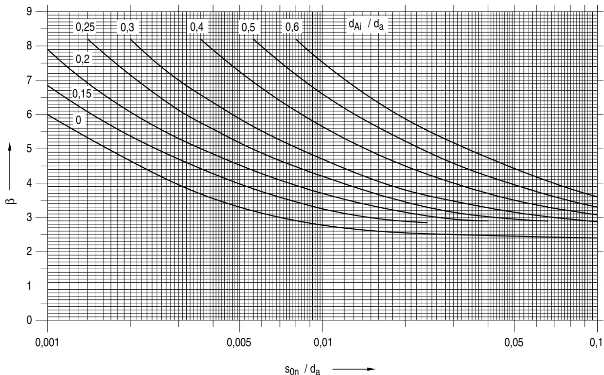
Bild A 2.5-3: Berechnungsbeiwerte \beta für gewölbte Böden in Klöppelform
