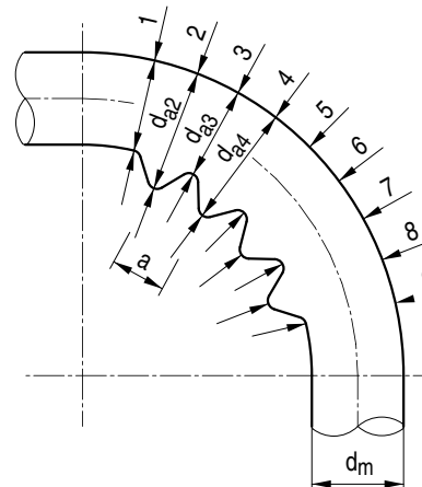
Bild A 4-1: Falten am Rohrbogen
