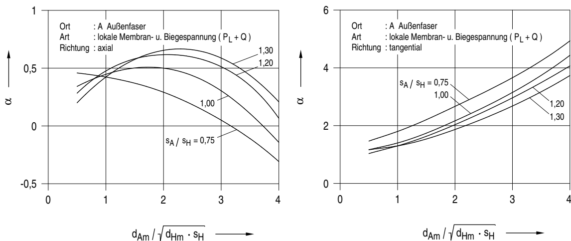
Bild 8.2-10: Spannungsbeiwert \alpha für Stutzen in zylindrischer Schale unter Innendruck
