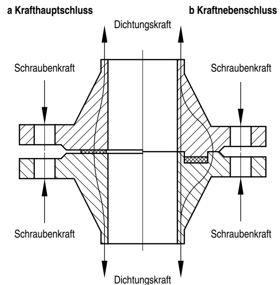
Bild A 2.8-1: Darstellung einer Flanschverbindung mit der Dichtung im KHS und im KNS (schematisch)
