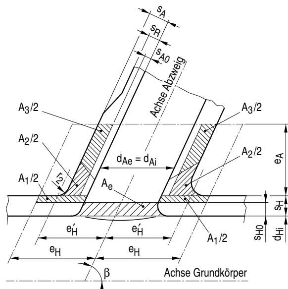
Bild A 2.7-8: Schräger zylindrischer Abzweig
