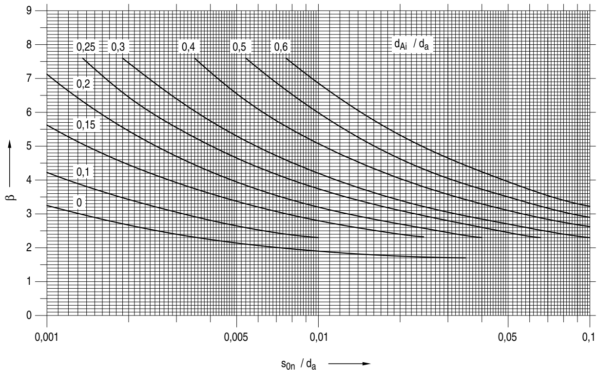
Bild A 2.5-4: Berechnungsbeiwerte \beta für gewölbte Böden in Korbbogenform
