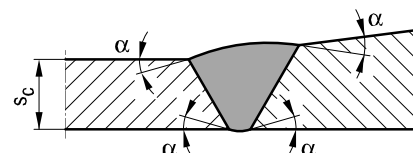
Bild 8.4-3: Zulässige Kontur der Schweißnaht
