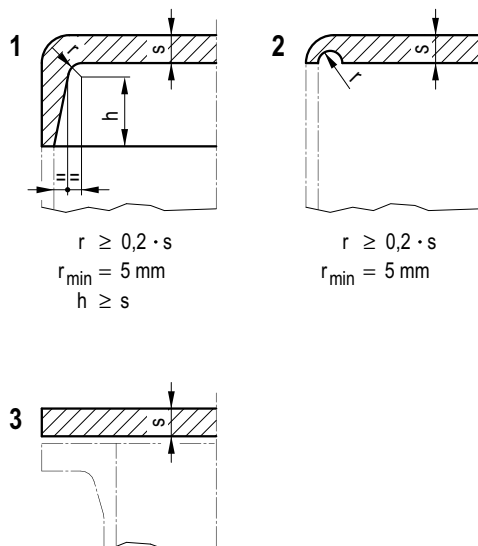
Bild 5.3-2: Deckel, Blindverschlüsse
