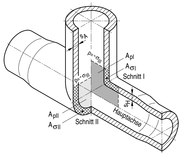
Bild A 3.1-5: Berechnungsschnitte für Gehäusekörper mit Abzweig
