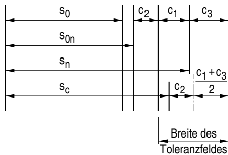
Bild 7.1-1: Wanddicken
