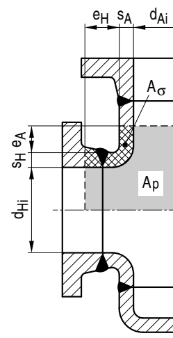
Bild A 3.1-12: Gehäusekörper
