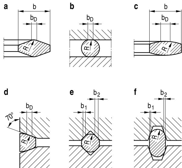
Bild A 2.10-3: Dichtungsprofile für Schmiegedichtungen
