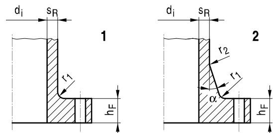
Bild 5.2-7: Vorschweißflansche
