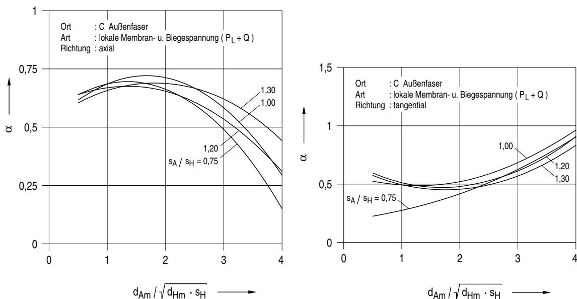
Bild 8.2-11: Spannungsbeiwert \alpha für Stutzen in zylindrischer Schale unter Innendruck
