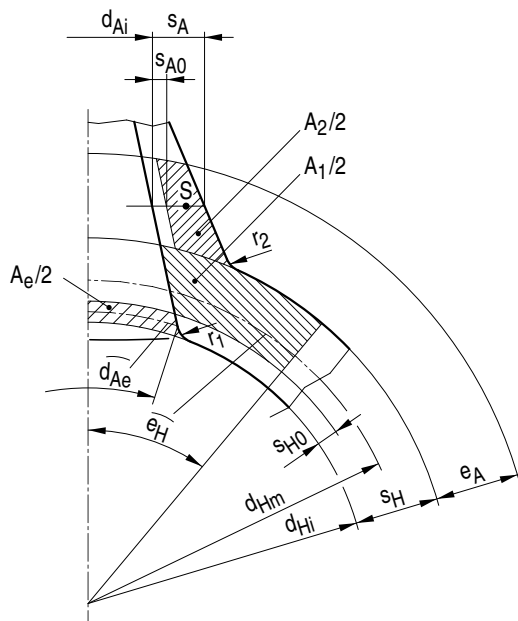
Bild A 2.7-11: Konischer Abzweig in einer Kugelschale
