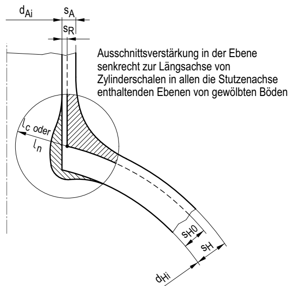
Bild A 2.7-12: Mittragende Zone
