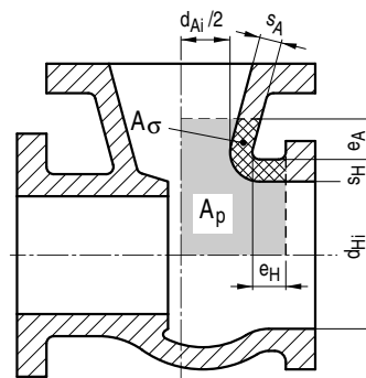
Bild A 3.1-9: Gehäusekörper in Eckform
