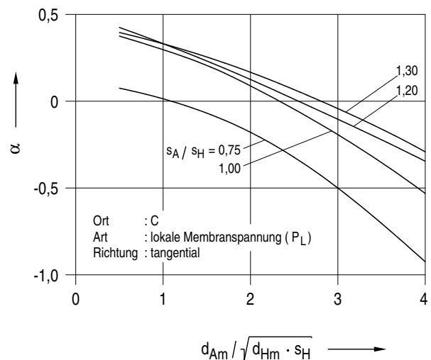
Bild 8.2-7: Spannungsbeiwert \alpha für Stutzen in zylindrischer Schale unter Innendruck
