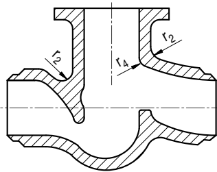
Bild 8.3-2: Ausrundungsradien
