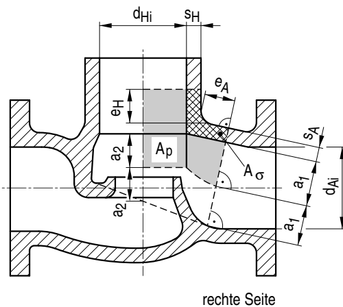
Bild A 3.1-7: Gehäusekörper
