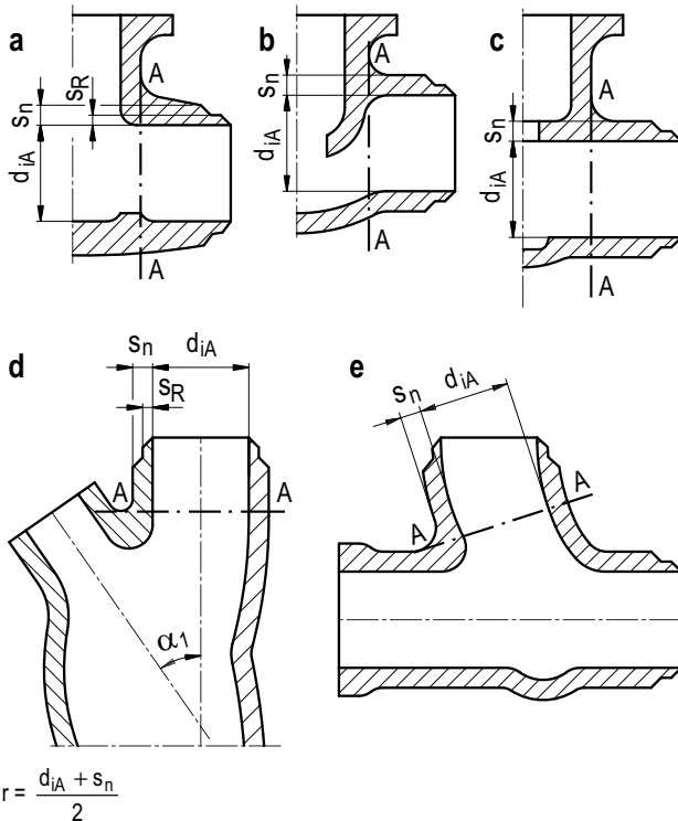
Bild 8.3-4: Maßgebende Schnitte an Armaturengehäusen
