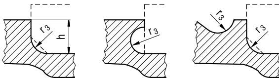
Bild 8.3-3: Zulässige Formen für Ausdrehungen
