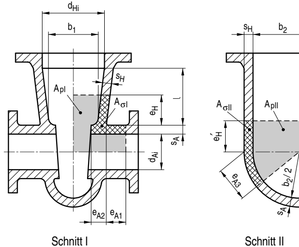
Bild A 3.1-6: Gehäusekörper
