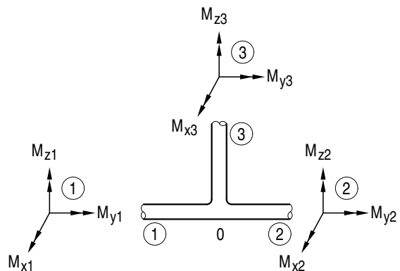
Bild 8.4-6: Bezeichnung der Momente am Abzweig
