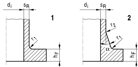
Bild 5.2-6: Vorschweißbünde
