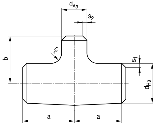
Bild A 4-8: Gepresstes Einschweiß-T-Stück
