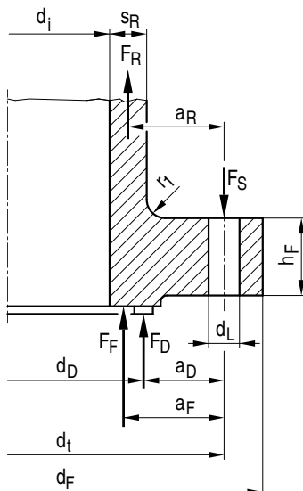
Bild A 2.9-4: Vorschweißflansch mit zylindrischem Ansatz
