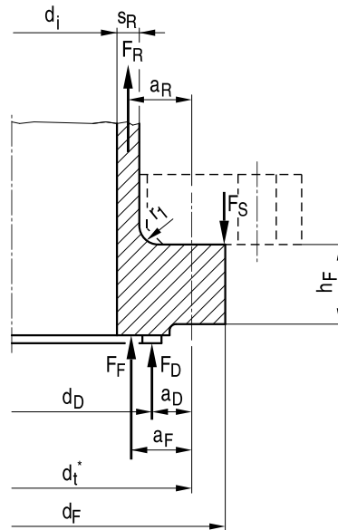
Bild A 2.9-5: Vorschweißbund mit zylindrischem Ansatz
