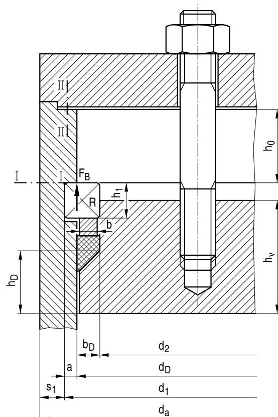
Bild A 3.4-1: Selbstdichtende Verschlüsse
