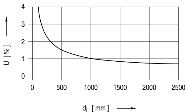
Bild 7.1-4: Unrundheiten
