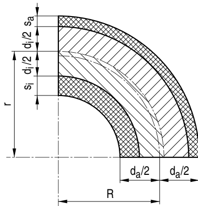
Bild A 4-2: Bezeichnungen am Rohrbogen
