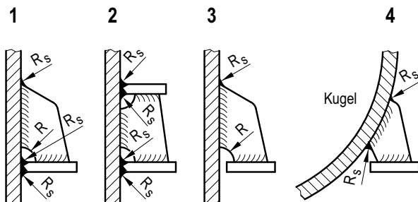
Bild 5.3-6: Beispiele für Komponentenstützkonstruktionen von stehenden Behältern mit Schmiederingen
