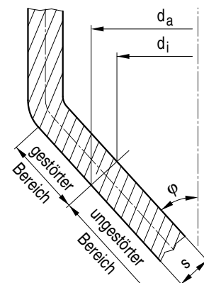
Bild A 2.4-2: Ungestörter Bereich einer Kegelschale
