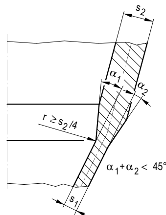
Bild 5.3-4: Gestaltung von Wanddickenübergängen
