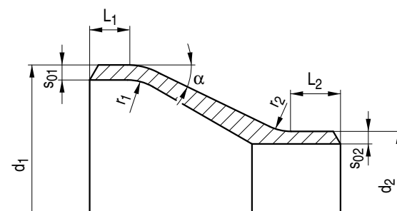
Bild 8.4-5: Konzentrisches Reduzierstück
