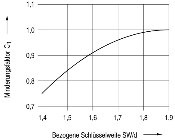
Bild A 2.8-6: Faktor C_1 zur Kennzeichnung der Verminderung der Abstreifkraft von Bolzen- und Muttergewinde infolge Mutteraufweitung
