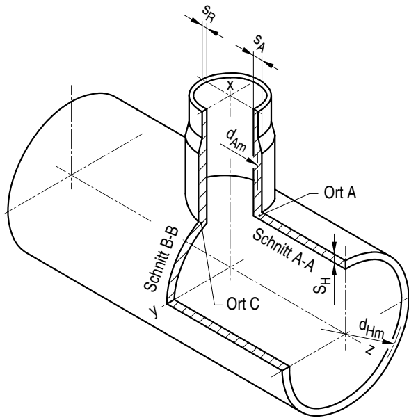
Bild 8.2-1: Stützen an zylindrischer Schale
