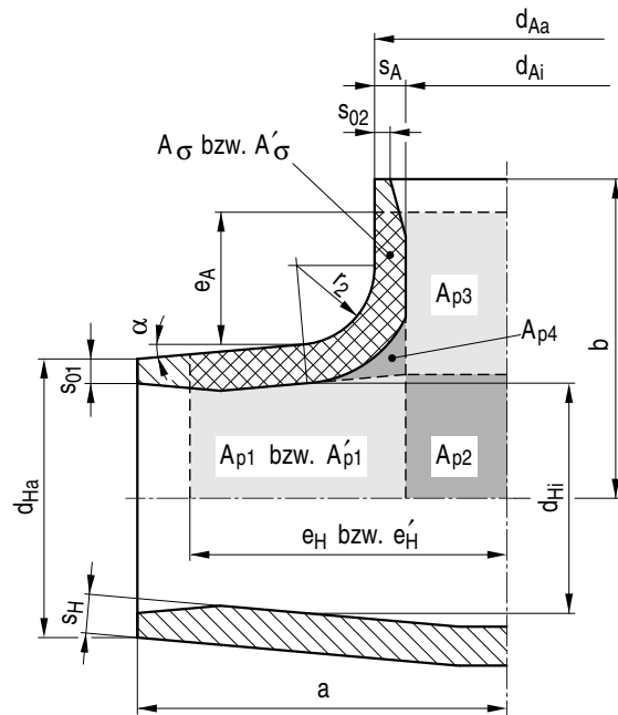
Bild A 4-9: Dimensionierungsflächen für Einschweiß-T-Stück
