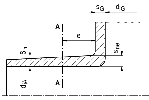
Bild 8.3-4: Maßgebende Schnitte an Armaturengehäusen
