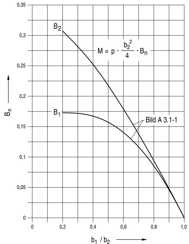
Bild A 3.1-2: Berechnungsbeiwert B_n für ovalförmige Querschnitte
