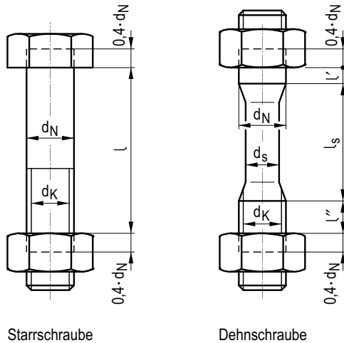
Starrschraube
