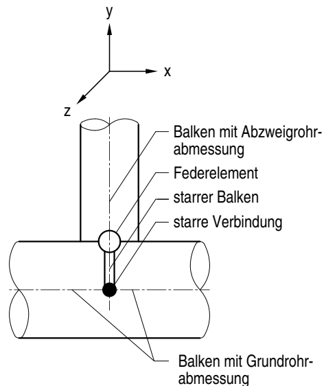
Bild 8.4-10: Modellierung von Abzweigen
