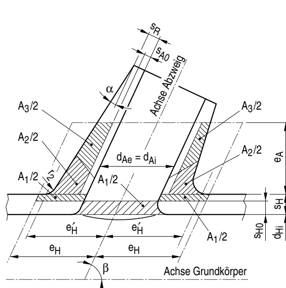
Bild A 2.7-9: Schräger konischer Abzweig
