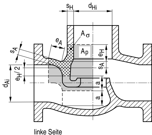
Bild A 3.1-8: Zylindrischer Gehäusekörper
