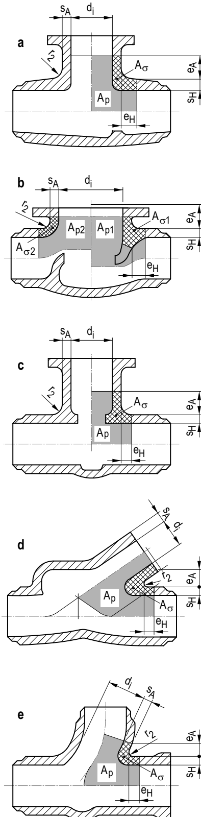
Bild 8.3-1: Flächenvergleichsmethode
