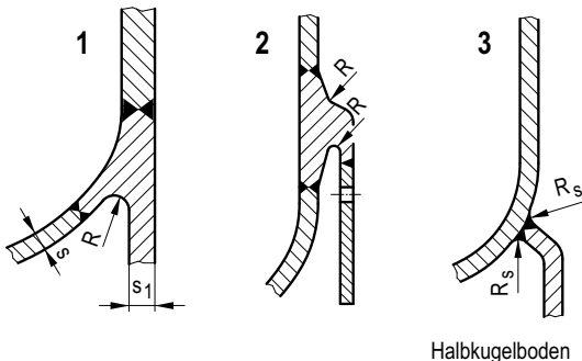
Bild 5.3-5: Beispiele für Komponentenstützkonstruktionen mit integralen Anschlüssen von stehend angeordneten Druckbehältern mit Standzarge
