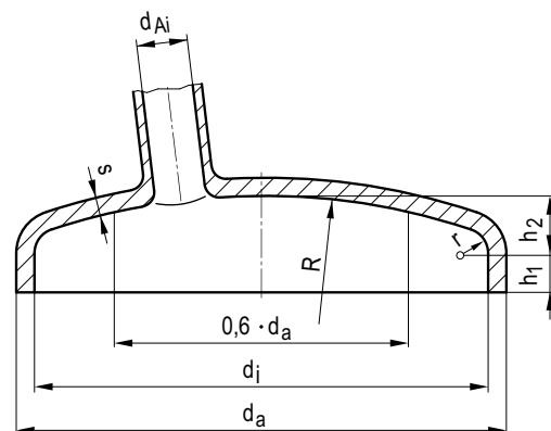
Bild A 2.5-2: Gewölbter Boden mit Ausschnitt
