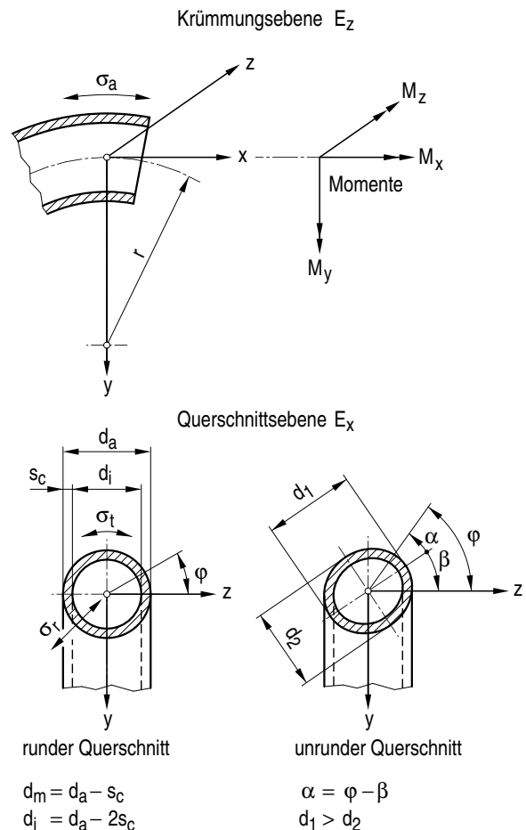
Bild 8.4-8: Bezeichnung am Rohrbogen für detaillierte Spannungsanalyse
