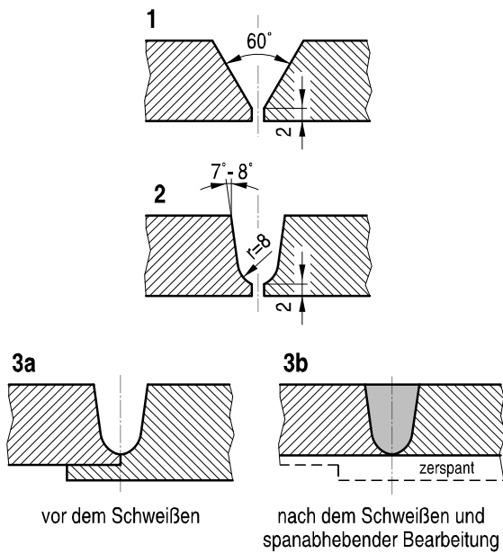
Bild 5.2-1: Beispiele für einseitig ausgeführte Stumpfnähte
