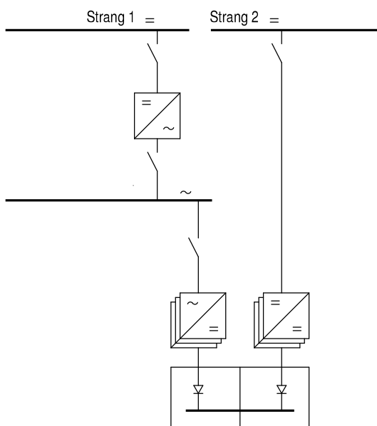
Bild 4-3: Beispiel eines Konzeptes mit redundanten Schalternetzteilkombinationen zur Versorgung von leittechnischen Einrichtungen
