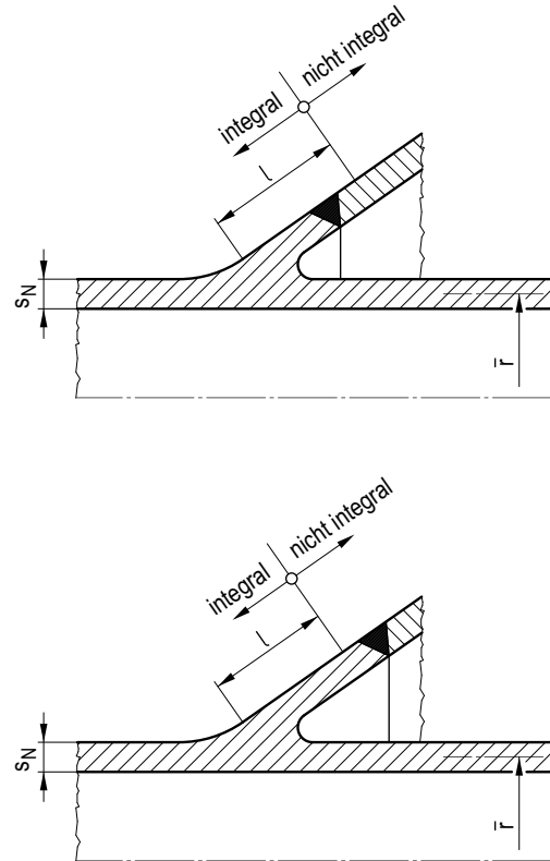
Bild 2-6: Beispiele für Stützkonstruktionen
