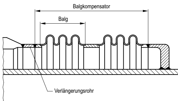
Bild 2-3: Balgkompensator
