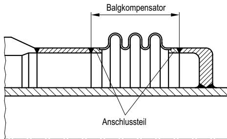
Bild 2-1: Anlussteil
