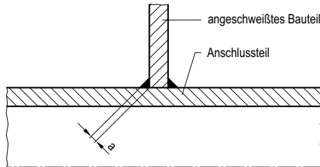
Bild A 4-2: Anschweißung
