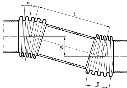
Bild A 5-1: Biegebalkenmodell
