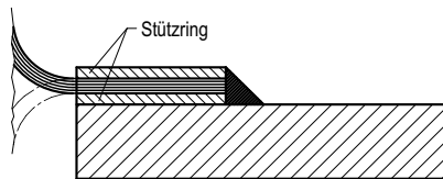
Bild 2-2: Stützring
