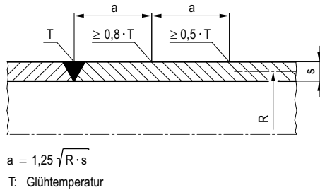
Bild B 4-1: Temperaturverlauf beim Spannungsarmglühen
