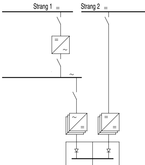
Bild 4-3: Beispiel eines Konzeptes mit redundanten Schaltnetzteilkombinationen zur Versorgung von leittechnischen Einrichtungen
