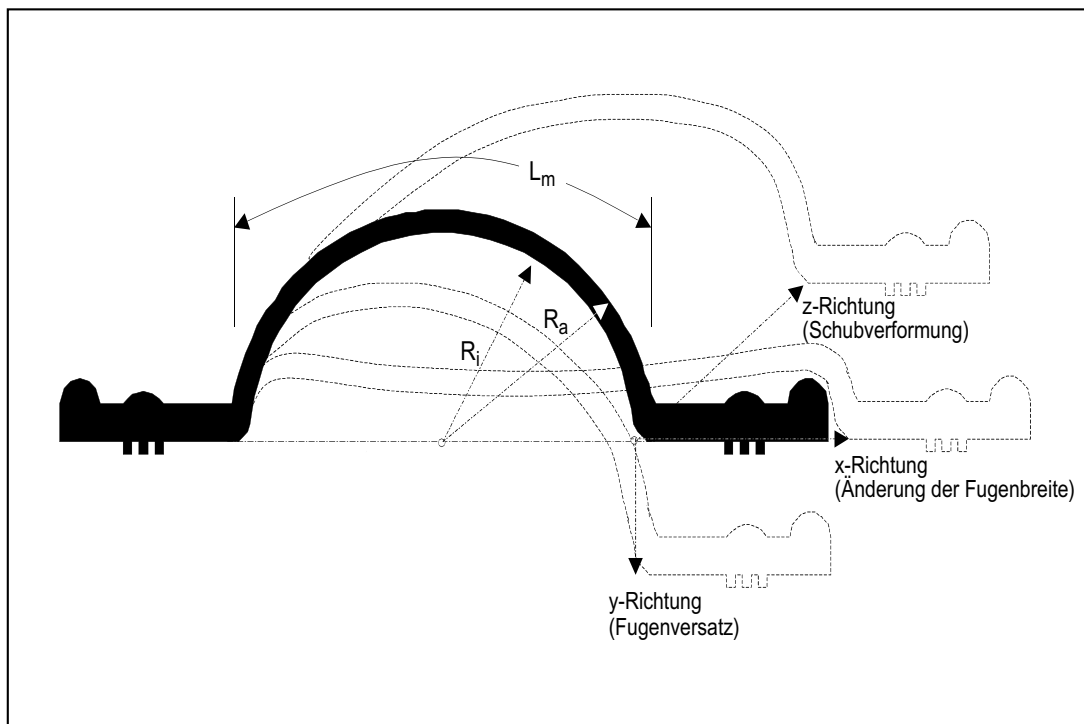
Bild 4-2: Beanspruchungsrichtungen eines Fugenbandes (Beispiel) mit Halbkreisschlaufe
